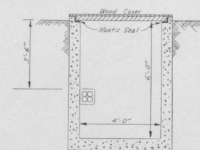
MANHOLE SECTION A-A SCALE: 1" = 2'
